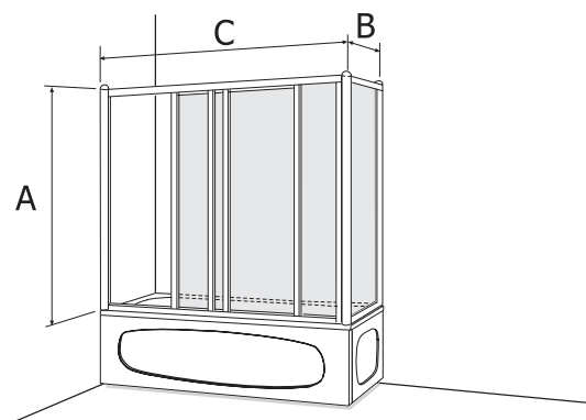
Drzwi rozsuwane do zabudowy wanien + ścianka boczna + profil A505882
