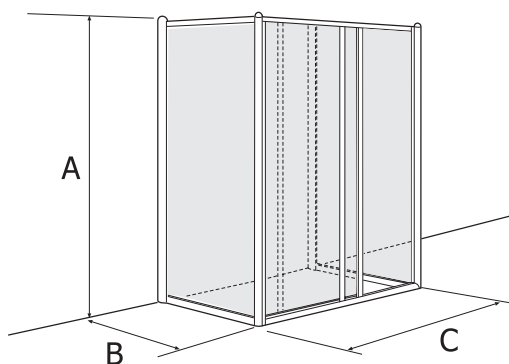
Drzwi rozsuwane + 2 ścianki + profil A505882
