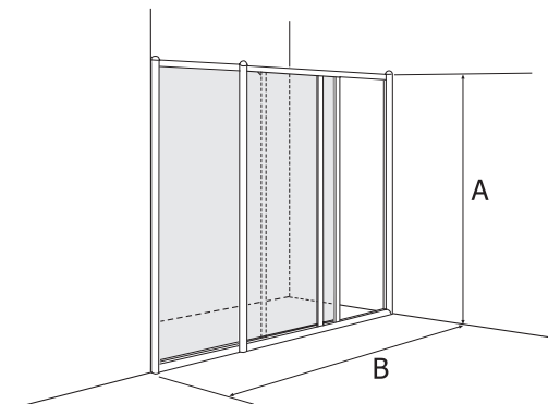
Zabudowa szerokiej wneki: drzwi rozsuwane + ścianka + profil A942582
